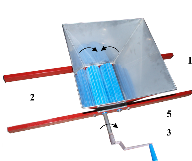
obr. 1 - drcení hroznů
